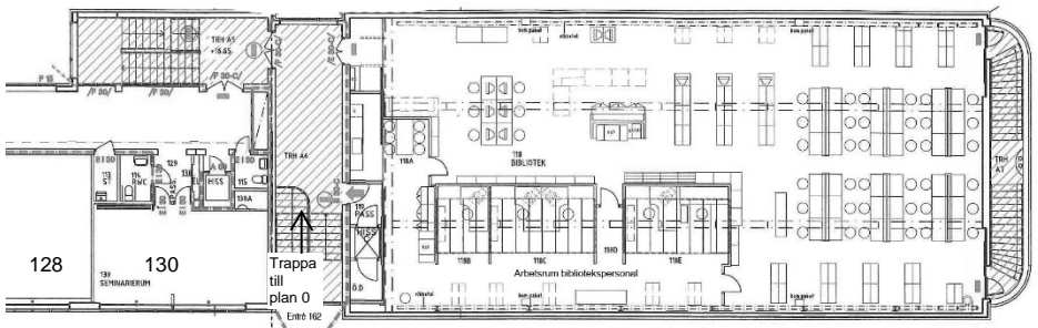
Biblioteket, Plan 1
