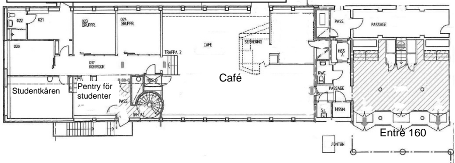
Plan 0 – entré, café och studentkåren
